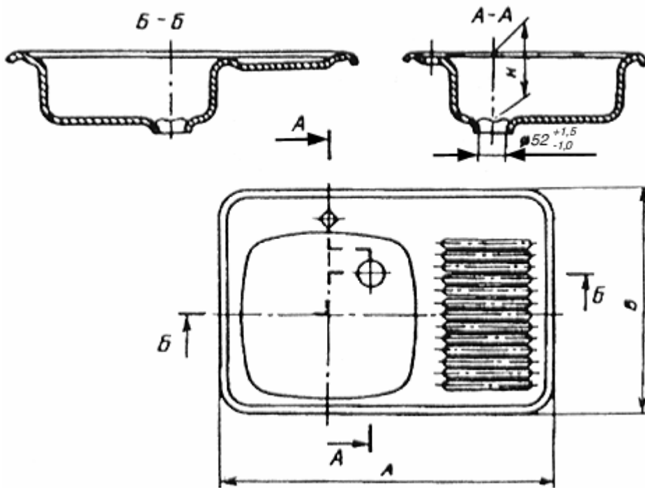
Рисунок 9 - Мойка стальная эмалированная с одной чашей со сливной полкой встраиваемая (тип МСВІІ)
