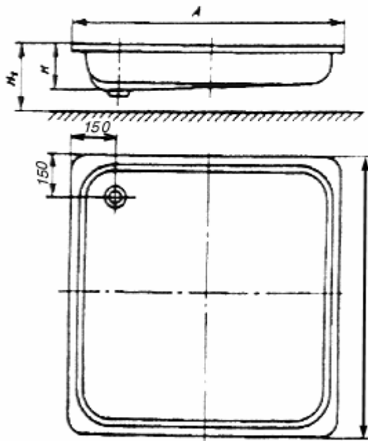
Рисунок 2 - Поддон мелкий стальной эмалированный (ПДСм)
