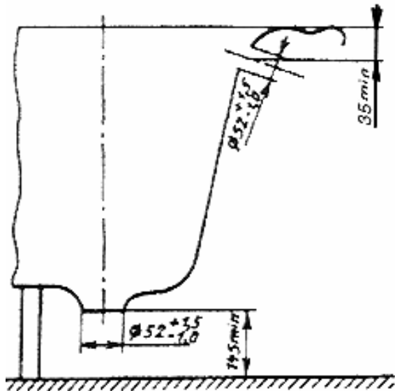
Рисунок 4 - Схема установки ванн и поддонов на опоры
