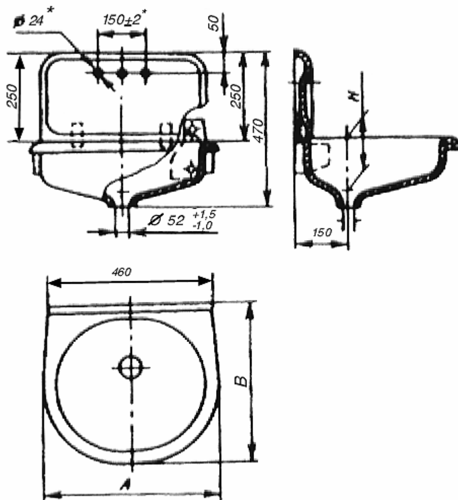
Рисунок 11 - Раковина стальная эмалированная (типы РСВ-1 и РСВ-2)
