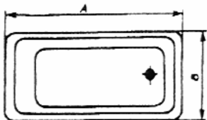
Рисунок 1 -Ванна стальная эмалированная (ВСт)
