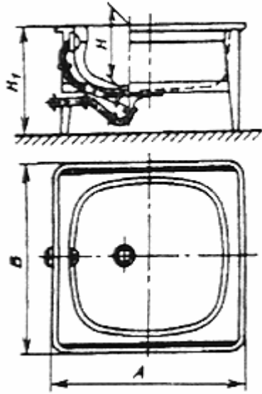
Рисунок 3 - Поддон глубокий стальной эмалированный (ПДСг)
